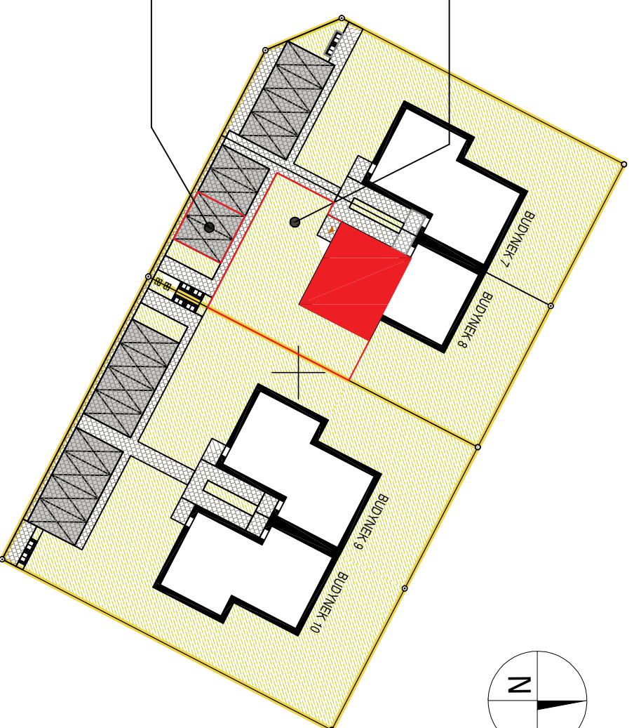
PLAN SYTUACYJNY
