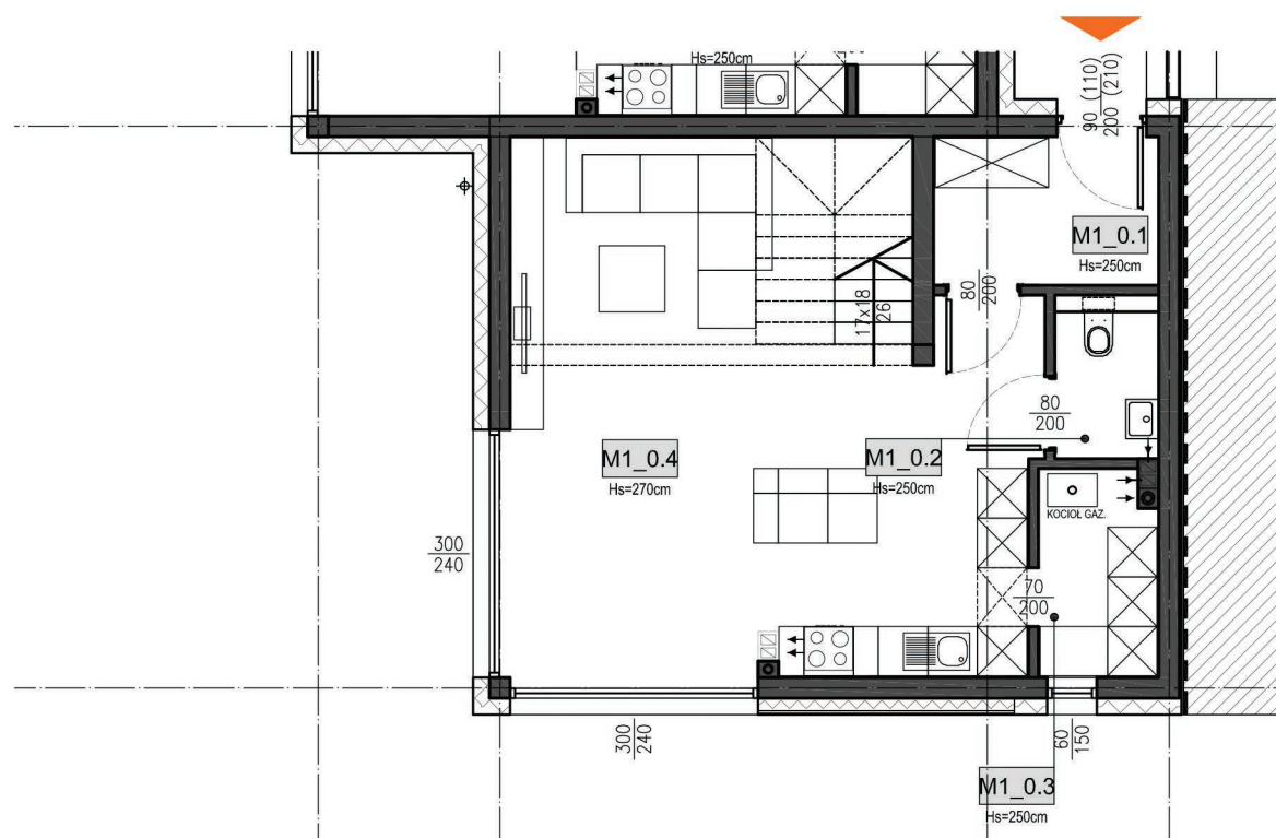
RZUT PARTERU
