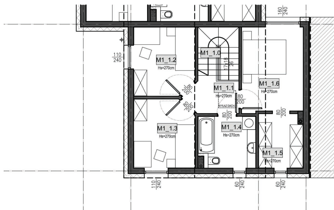
RZUT PIĘTRA
